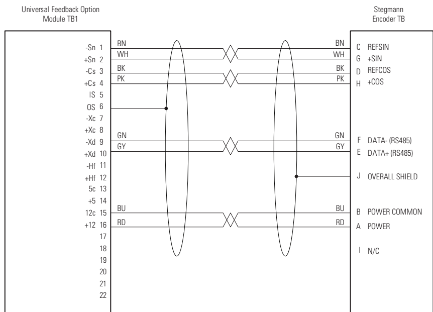
图 71 - Stegmann 旋转式编码器通过带有 10 针 MS 式连接器的屏蔽式双绞线电缆进行连接
