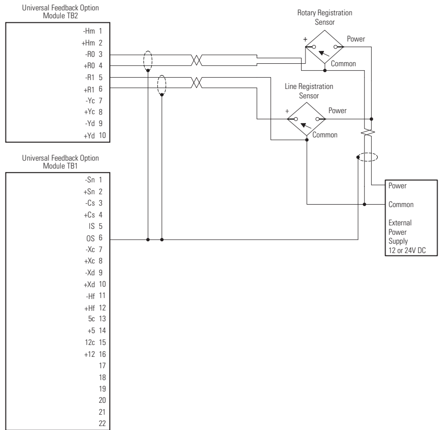
图 74 - 定位传感器
