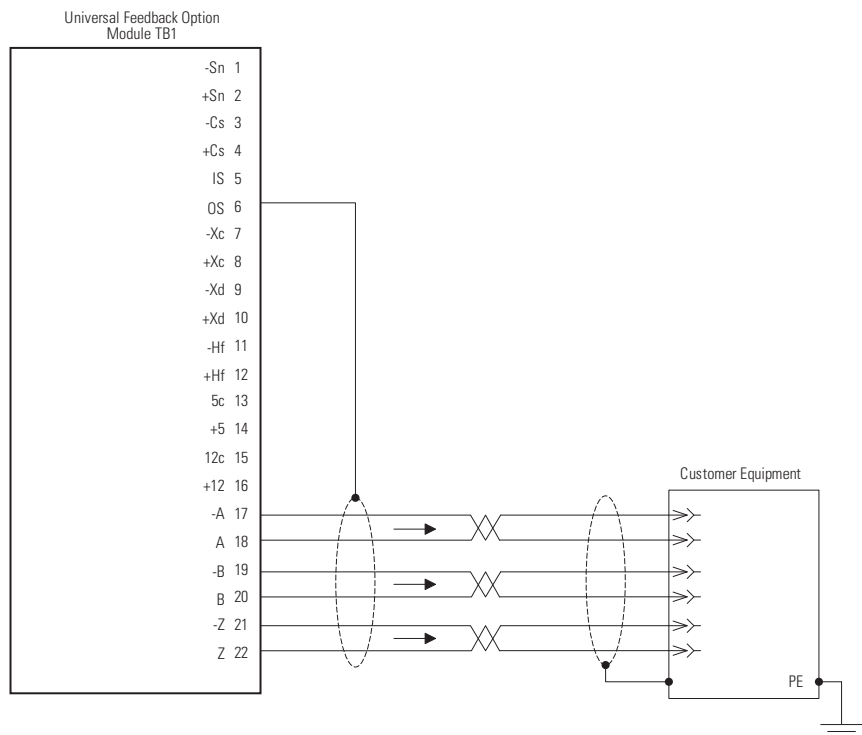
图 75 - 模拟的增量型编码器输出 \
