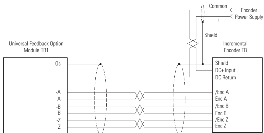
图 77 - 带具有外部电源的 Z 通道的差分双通道
