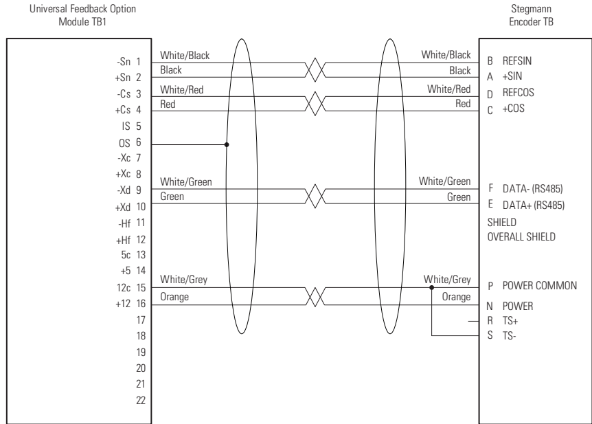
图 67 - HPK 系列电机和 Stegmann 旋转式或普通旋转式编码器通过 2090-XXNFMF-SXX 电缆进行连接
