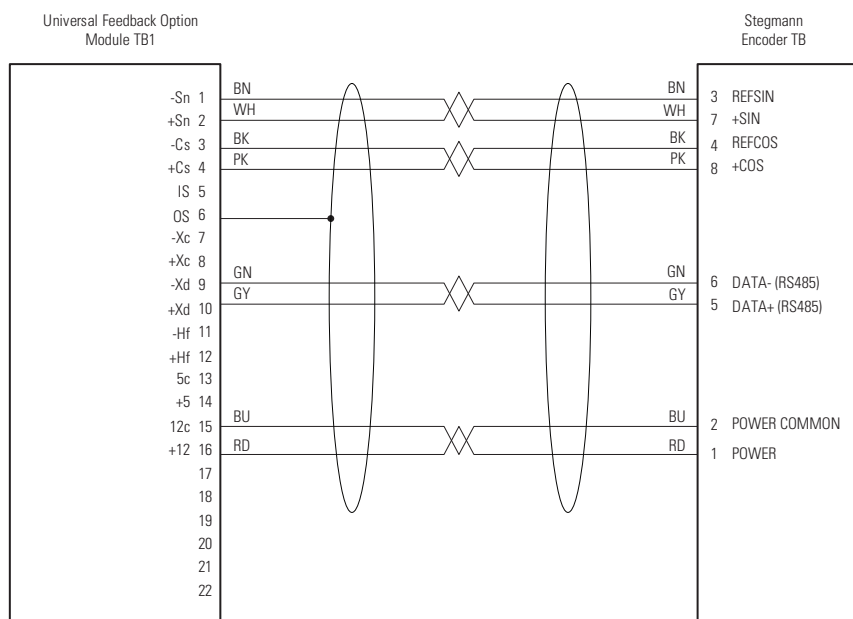
图 69 - Stegmann 旋转式编码器通过预连接的屏蔽式双绞线电缆进行连接
