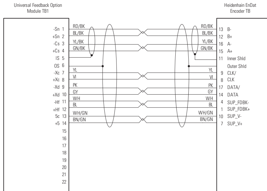
图 59 - 带内部电源的 Heidenhain EnDat 角度编码器
