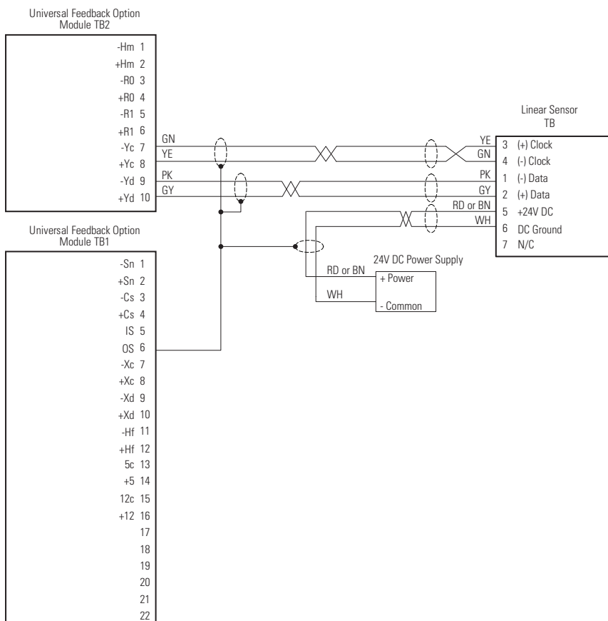
图 73 - 带有 MDI RG 连接器或 P 整体式电缆的线性传感器
