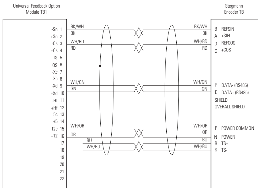
图 65 - 460V MP 系列或 Allen-Bradley 1326AB 系列电机和 Stegmann 旋转式或普通旋转式编码器通过 2090-XXNFMF-SXX 或 2090-XXNFMP-SXX 电缆进行连接。 HPK 系列电机通过 2090-XXNFMF-SXX 电缆进行连接
