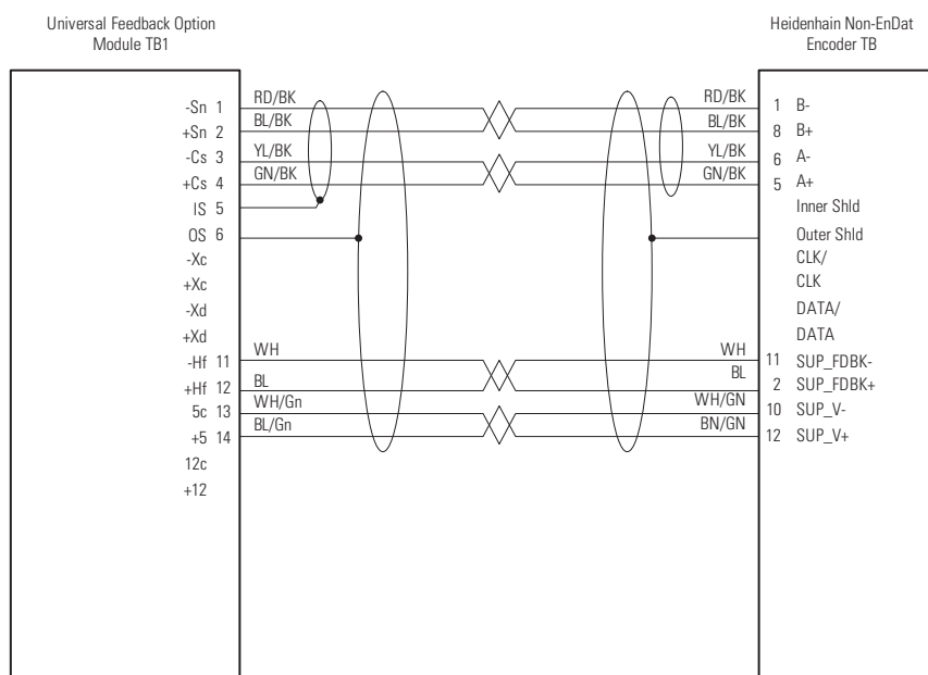
图 61 - 带内部电源的 Heidenhain 非 EnDat 旋转编码器
