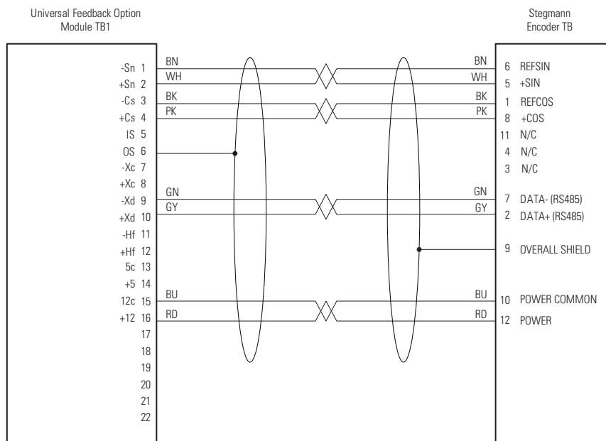
图 72 - Stegmann 旋转式编码器通过带有 12 针 DIN 式连接器的屏蔽式双绞线电缆进行连接
