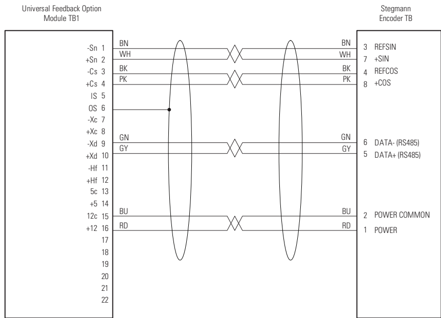
图 70 - Stegmann 旋转式编码器通过带有 8 针 Berg 式连接器的屏蔽式双绞线电缆进行连接
