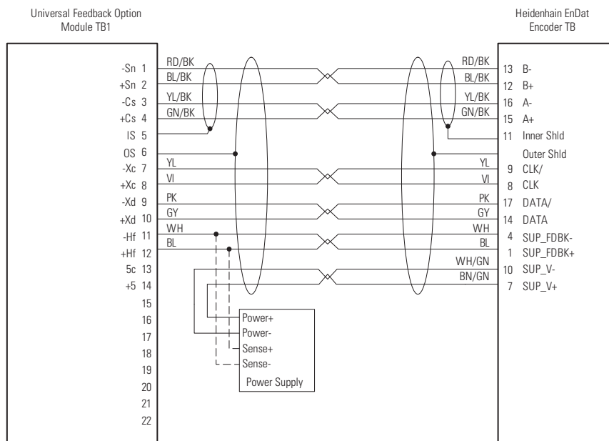
图 60 - 带外部电源的 Heidenhain EnDat 角度编码器
