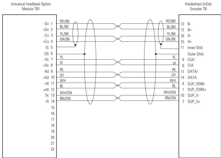
图 62 - 带内部电源的 Heidenhain EnDat 旋转编码器 (ECN 412 EnDat01)
