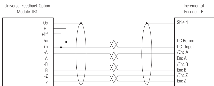
图 76 - 带具有 5V 内部电源的 Z 通道的差分双通道
