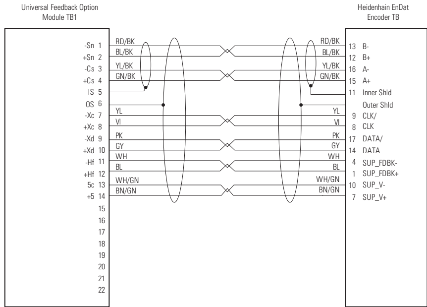
图 63 - 带内部电源的 Heidenhain EnDat 旋转编码器 (ECN 412 EnDat01)
