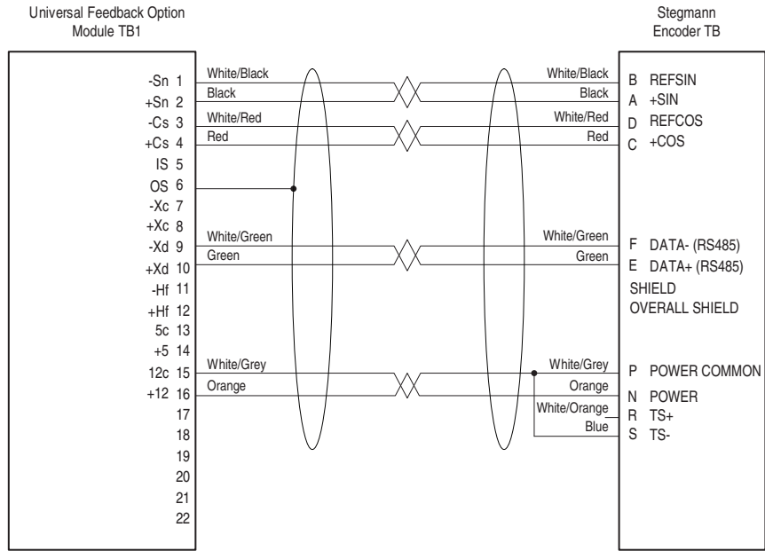
图 66 - 460V MP 系列电机和 Stegmann 旋转式或普通旋转式编码器通过 2090-CFBM7XX-CDAFX 电缆进行连接
