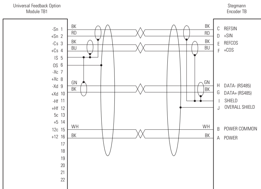
图 68 - Stegmann 旋转式编码器通过 1326-CECU-XXL-XXX 电缆进行连接
